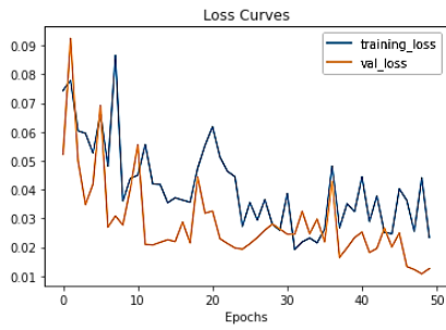
(d) InceptionV3
