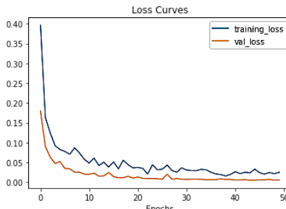
(e) Xception
