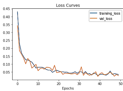
(g) NASNetMobile
