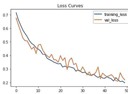
(h) VGG19
